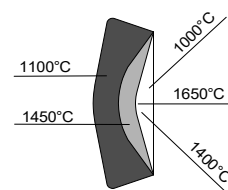
Flammenbild und Temperaturverteilung
