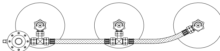
Dreiflaschenanlage
