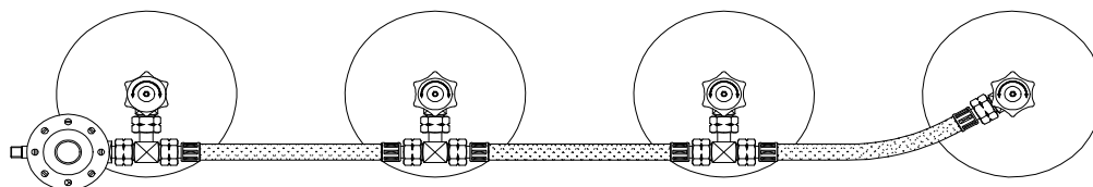
Vierflaschenanlage
